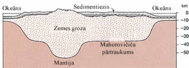
7. attēls. Kalniem ir dziļas saknes zem zemes virsmas. ( Earth , Press and Siever, p. 413.)
