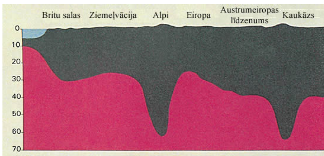
8. attēls. Shematisks griezum. Kalni, gluži kā tapas, ir ar dziļām saknēm iestiprināti zemē. ( Anatomy of the Earth , Cailleux, p. 220.)
